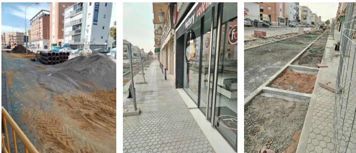
En las fotografías se muestra el proceso de las obras, donde ya se aprecia el nuevo acerado, el carril bici y la zona para plantar los árboles.
